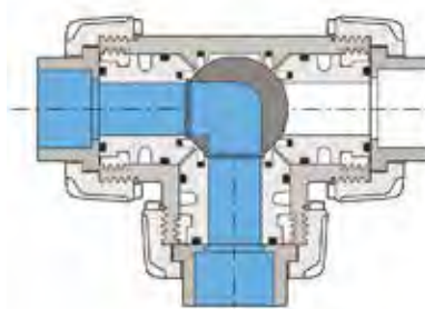
E - Valvola sfera a L: 0°/270° - Smistamento
